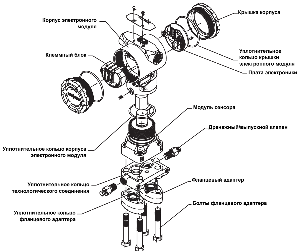
Рис.А-1. Схема запасных частей
