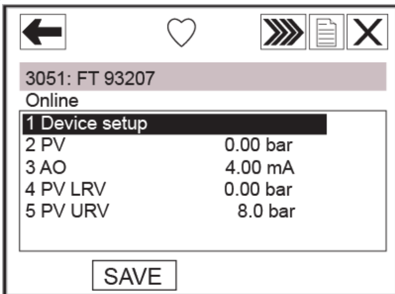
Рис. 3-4. Индикаторная панель устройства
