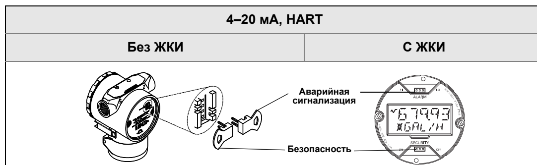
Рис. 2-13. Плата электроники
