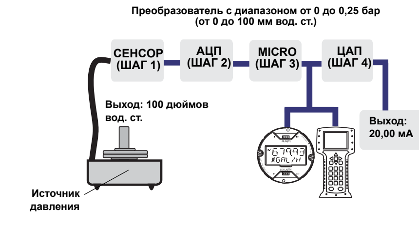
Рис. 4-1. Схема обмена данными с преобразователем с возможностями калибровки
